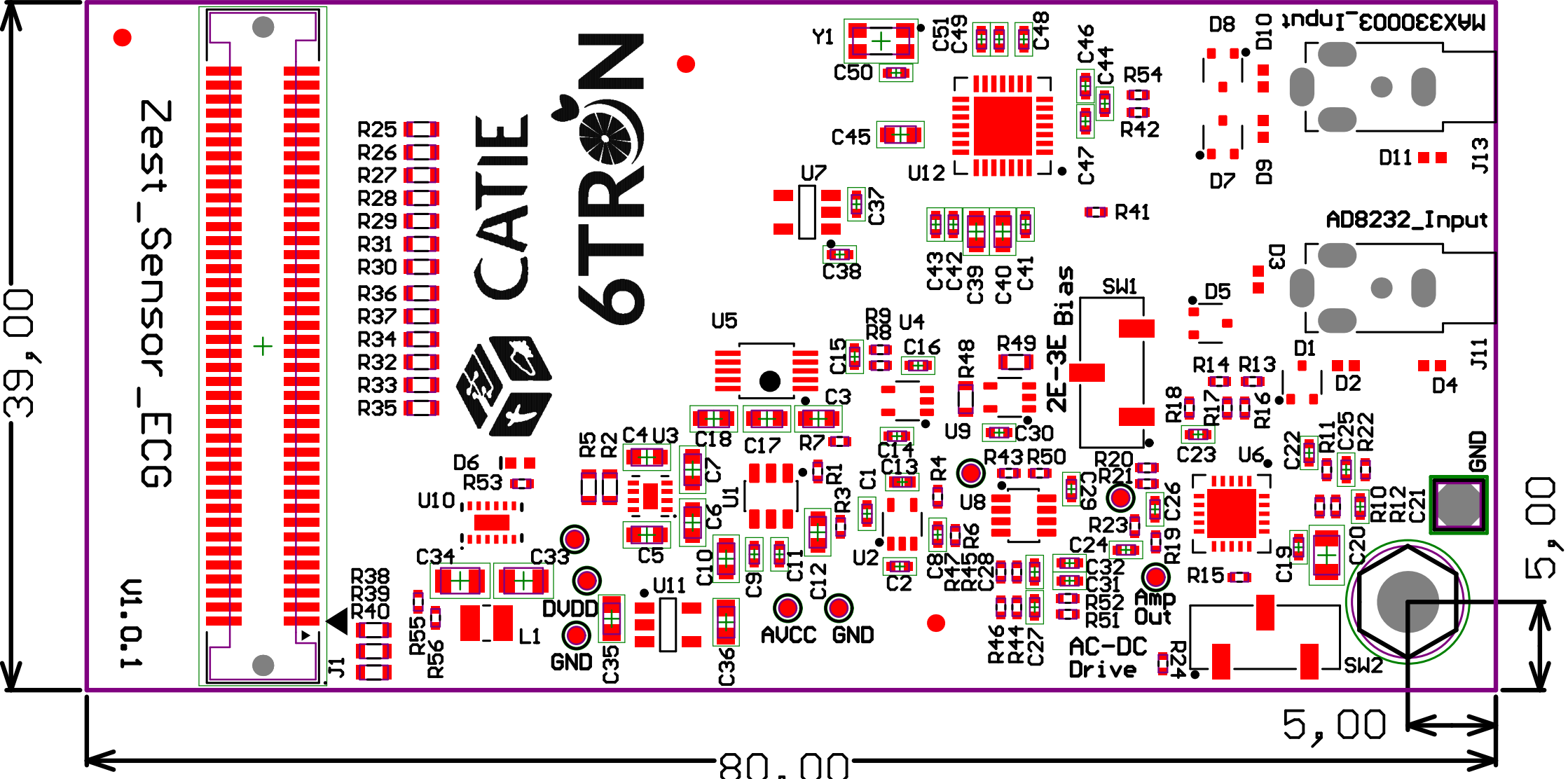
Top Overlay
